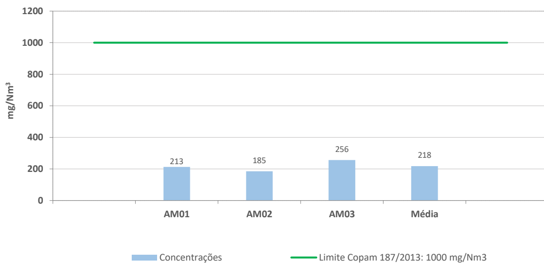
Gráfico 02 - CHAMINÉ DA CALDEIRA DEDINE CBC B 14. B03 - Óxidos de Nitrogênio (NOx)
