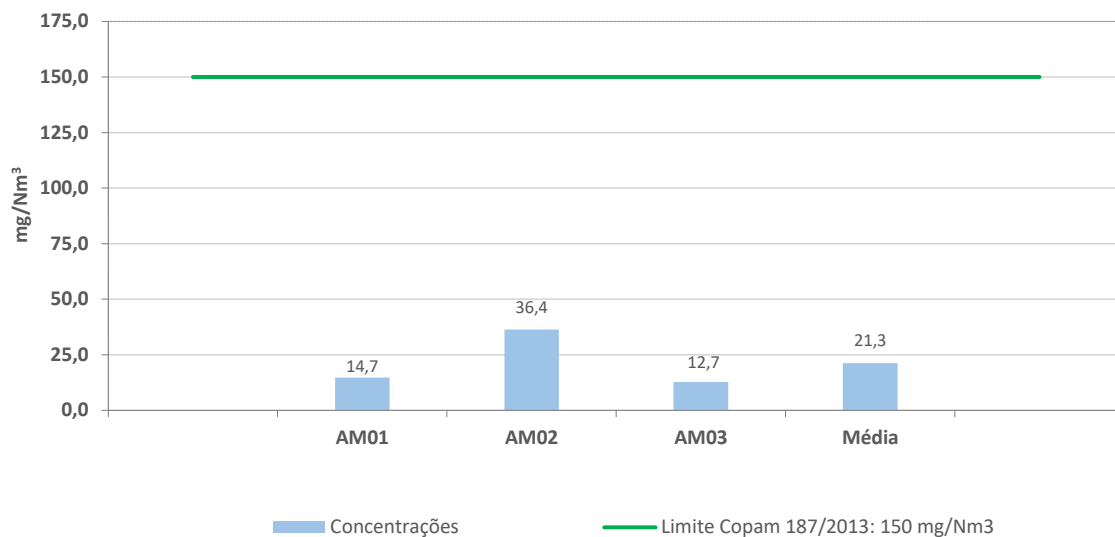
Gráfico 01 - CHAMINÉ DA CALDEIRA DEDINE CBC B 14. B03 - Material Particulado (MP)
